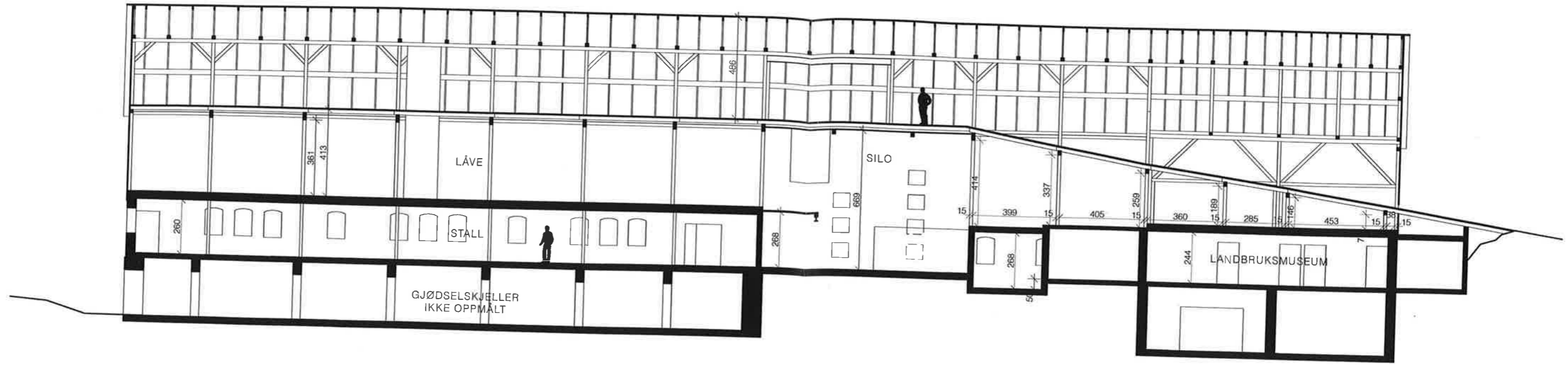
Snitt A-A
