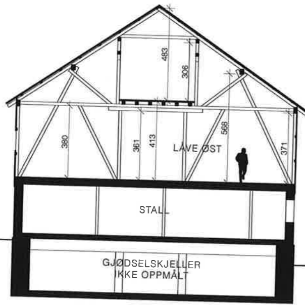
Snitt B-B
