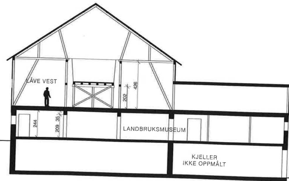
Snitt C-C
